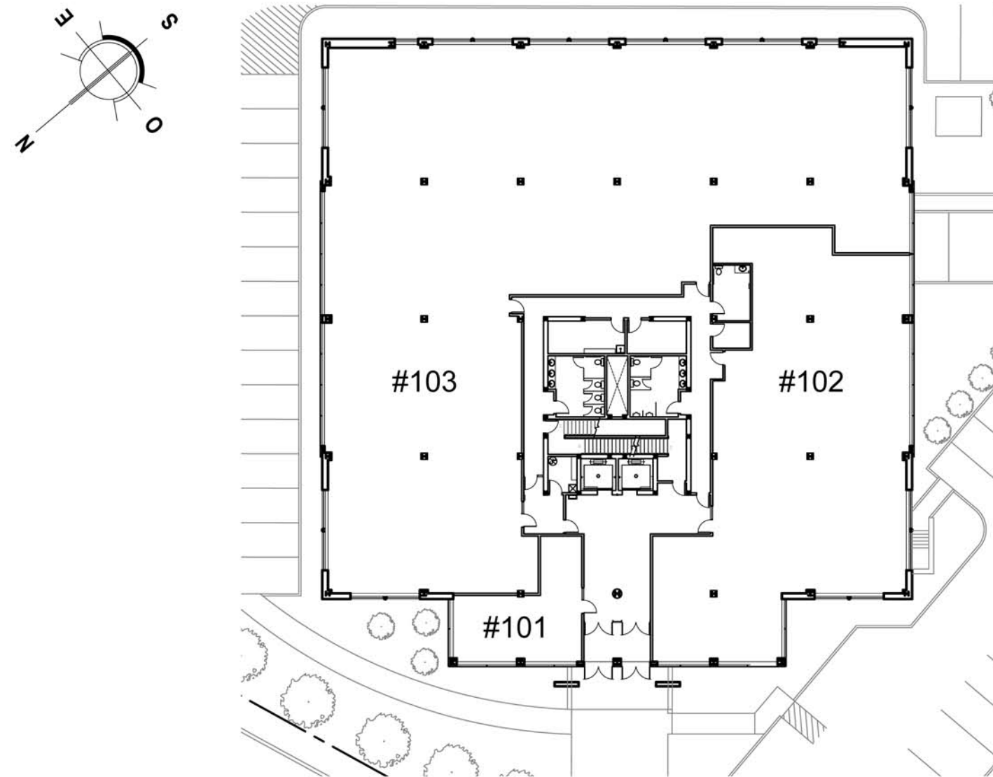
REZ-DE-CHAUSSÉE
