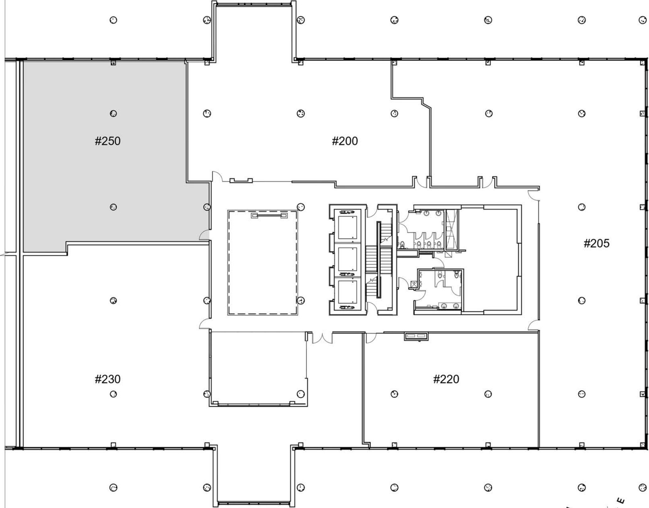
2ième ÉTAGE
